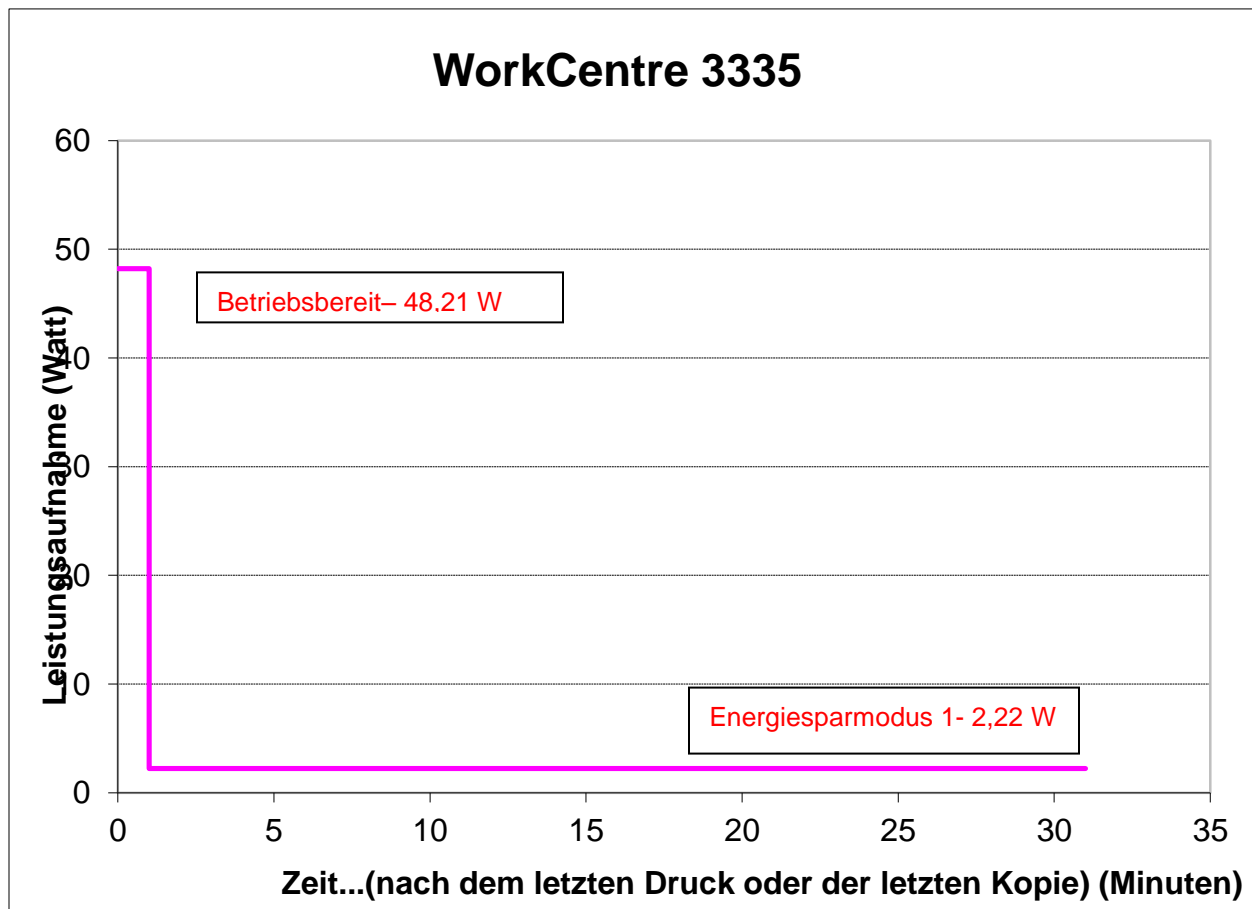
Darstellung 1 – Leistungs-Profil
